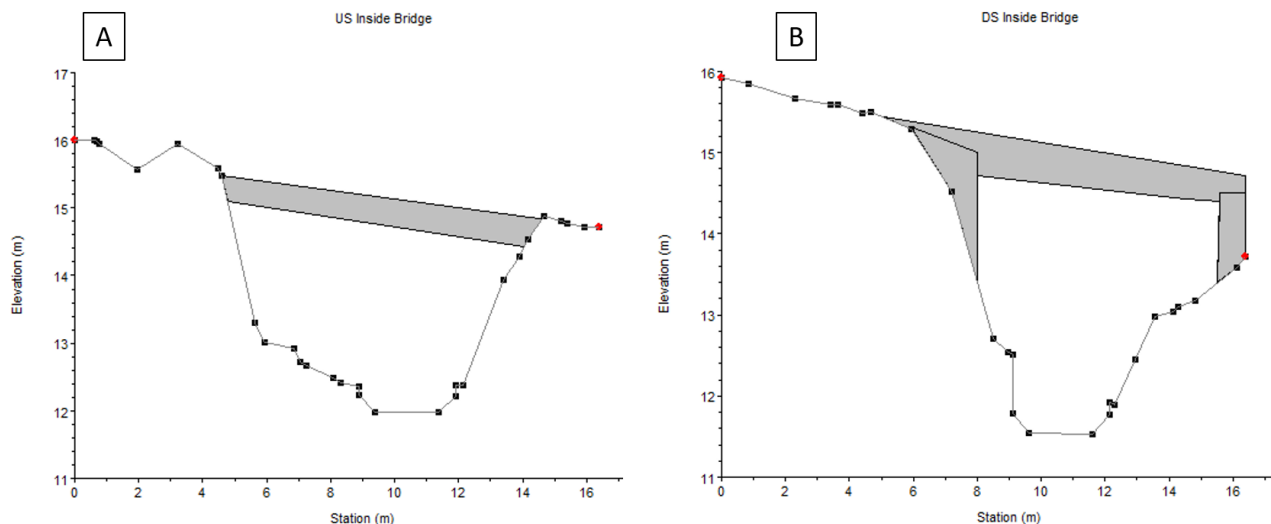
Figur 22: Tverrsnitt av bru B8, ved A) oppstrøms og B) nedstrøms side
