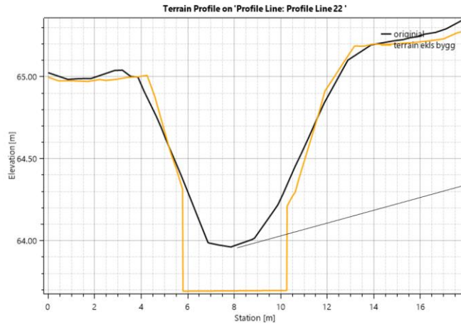
Figur 3: Terrengendring i elveløp mellom bru B2 og B3
