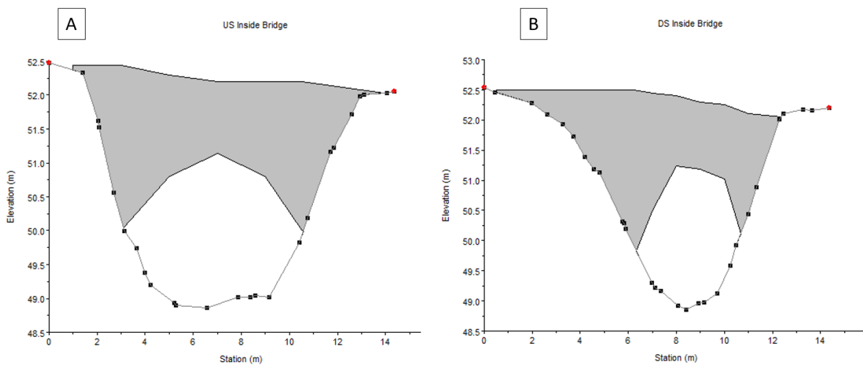
Figur 17: Tverrsnitt av bru B6 fra HEC-RAS av A) oppstrøms og B) nedstrøms side
