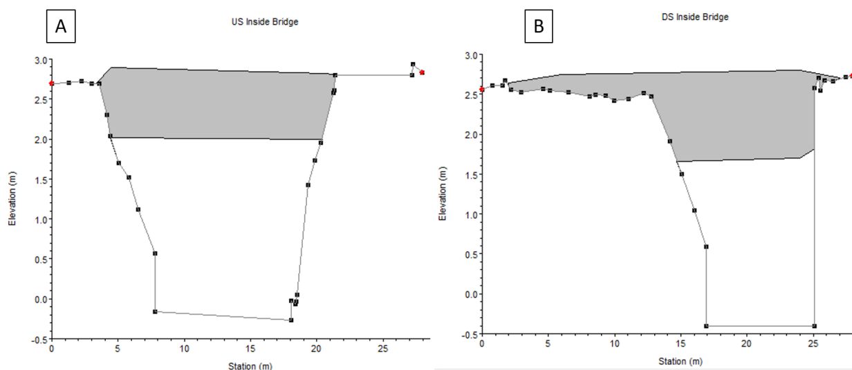
Figur 26: Tverrsnitt fra bru B9 ved A) oppstrøms og B) nedstrøms side
