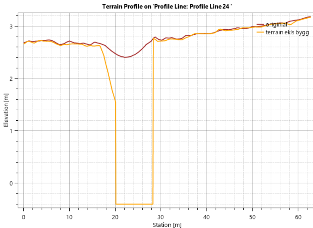
Figur 27: Senkning av terrenget under bru B9 basert på oppmåling av bruene og elveløpet.
