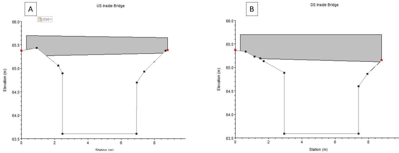
Figur 7: A) Oppstrøms og B) nedstrøms tverrsnitt av bru B3
