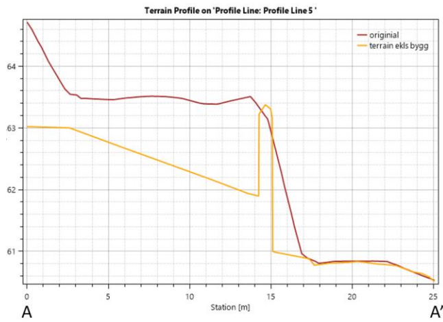
Figur 11: Terrengendring mellom bru B4 og dam Porkegjel
