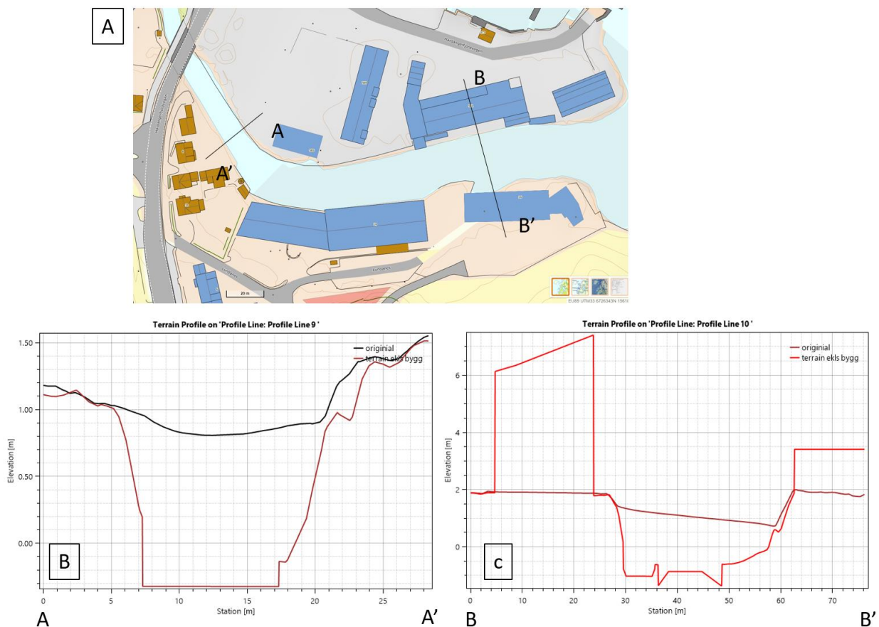
Figur 29: To tverrsnitt nedstrøms av bru B9 som viser senkning av terreng i elveløpet. I C) Bygninger er inkludert i terrengmodellen.
