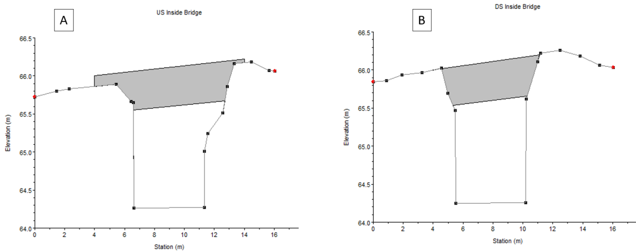
Figur 5: Tverrsnitt av bru B2 av A) oppstrøms og B) nedstrøms side
