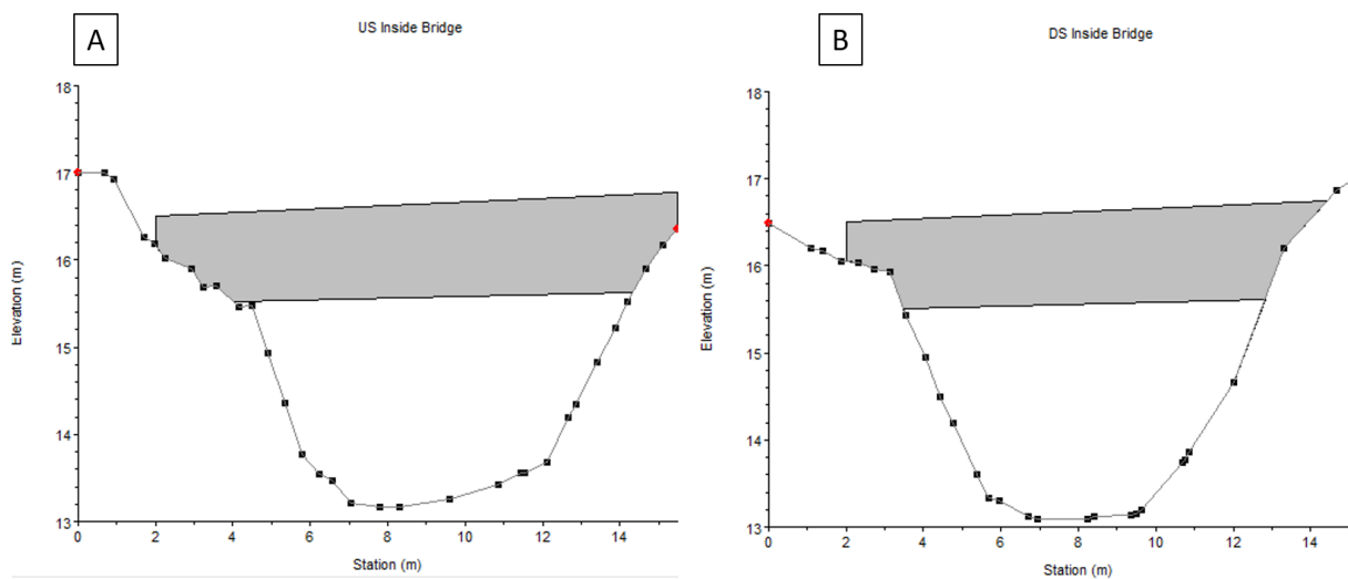
Figur 20: Tverrsnitt av rørgate, ved A) oppstrøms og B) nedstrøms side
