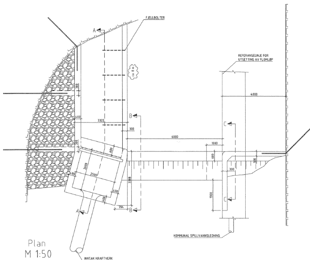
Figur 14: Utklipp fra tegning (Porkegjel Inntaksdam 5-6-2007).
