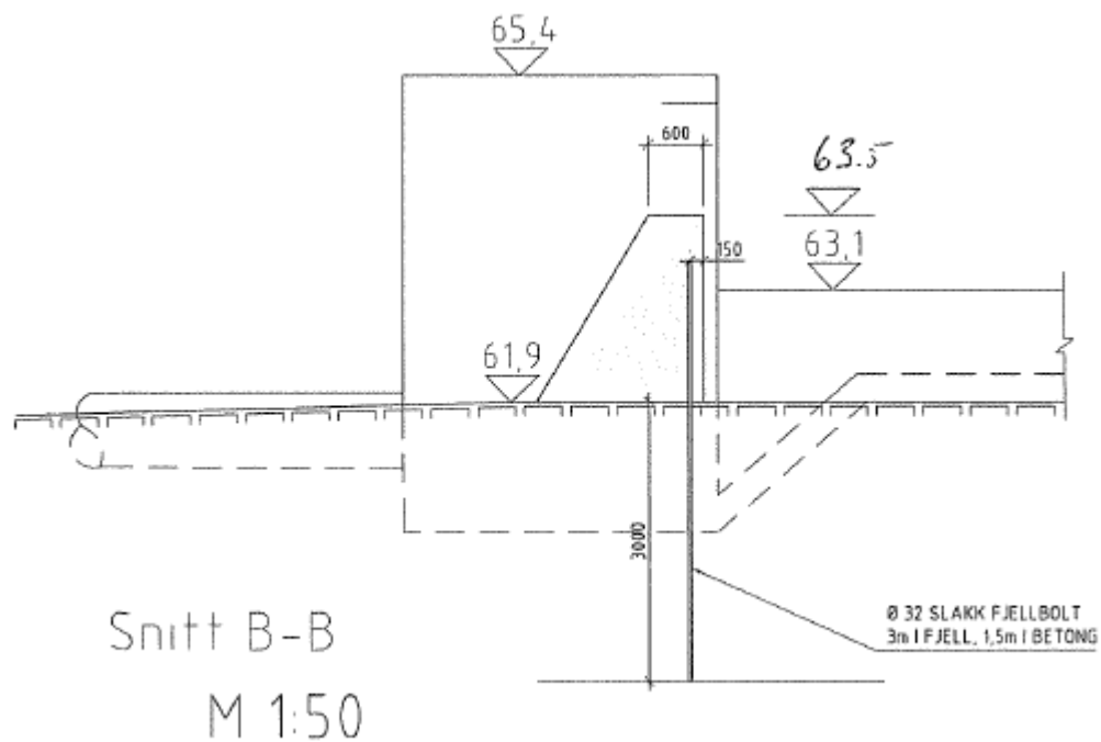
Figur 15: Utklipp fra tegning (Porkegjel Inntaksdam 5-6-2007).
