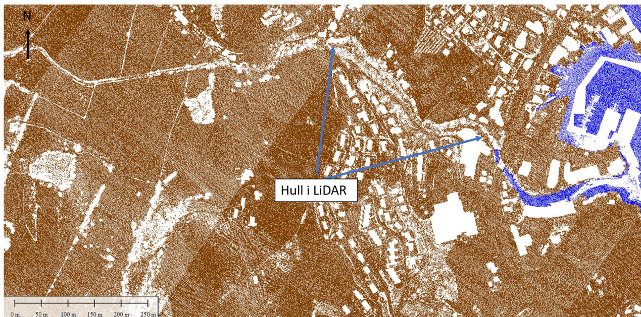
Figur 7: Hull i LiDAR data (hvitte områder) etter filtrering for bakkepunkter (brune punkter).
