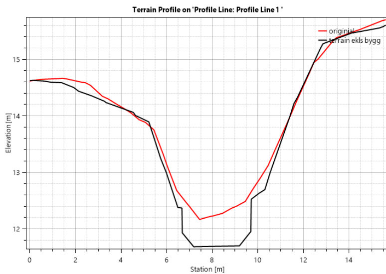
Figur 23: Terrengendring under bru B8
