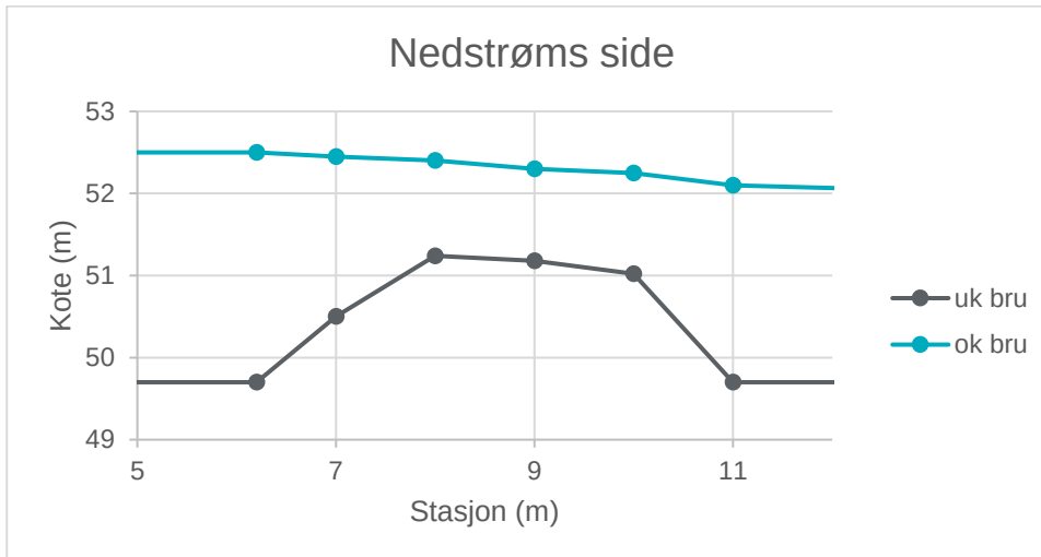
Figur 18: Nedstrøms tverrsnitt av bru B6
