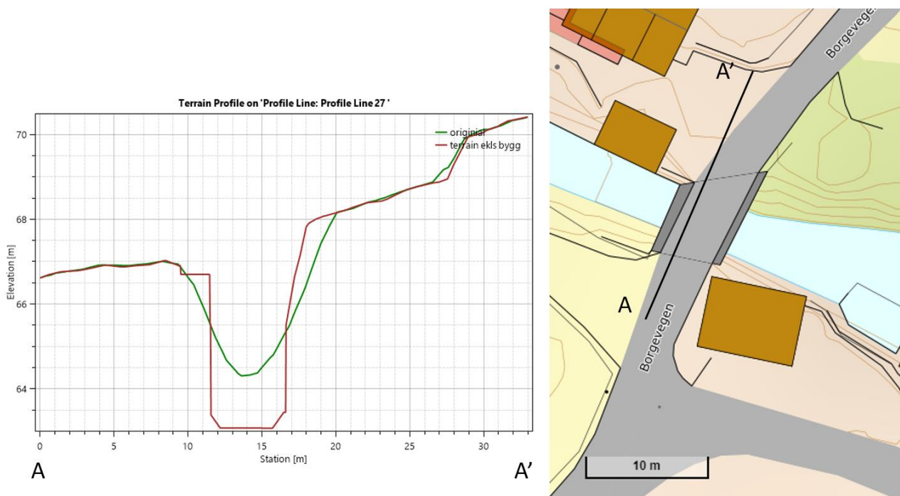
Figur 10: Terrengendring på bru B4, landkar på vestsiden er hevet og elvebunn er senket
