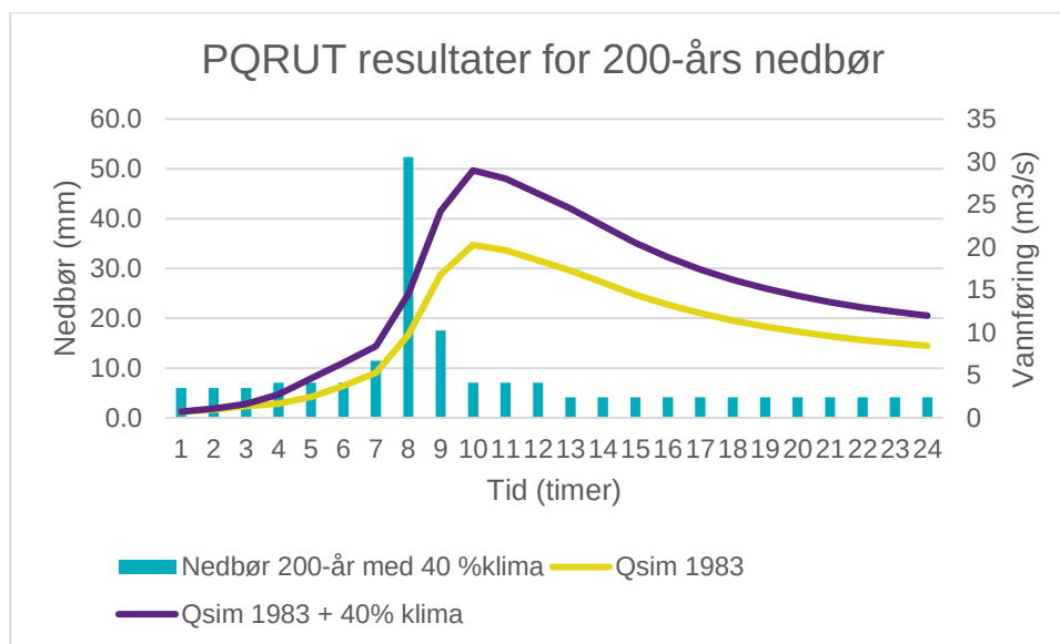
Figur 4: Resultater fra PQRUT beregninger.
