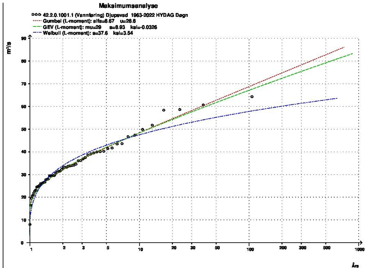
Figur 3: Ekstremver dianalyse resultat fra Hydra 2 for nedbørfelt til Djupevad
