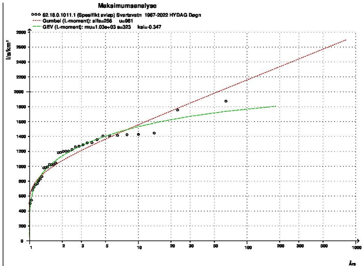
Figur 2: Ekstremver dianalyse resultat fra Hydra 2 til nedbørfelt til Svartavatn
