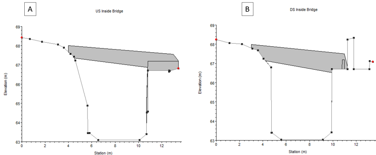
Figur 9: Tverrsnitt av bru B4 av A) oppstrøms og B) nedstrøms side
