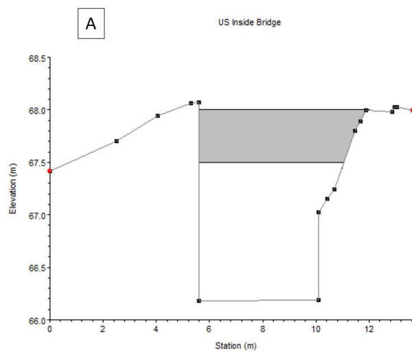
Figur 4: Tverrsnitt av bru B1 av A) oppstrøms side og B) nedstrøms
