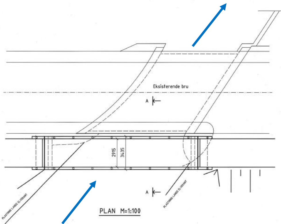
Figur 25: Utklipp av tegning av utvidelse av bruene i 1991 (tegningsnr. 2877-K01), underkant av utklipp er oppstrøms side.
